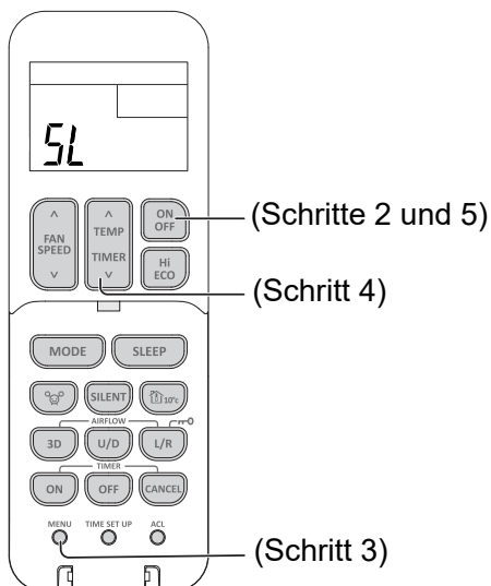
Abbildung 13: Infrarotfernbedienung für Wandgeräte SRK-ZTL-W
