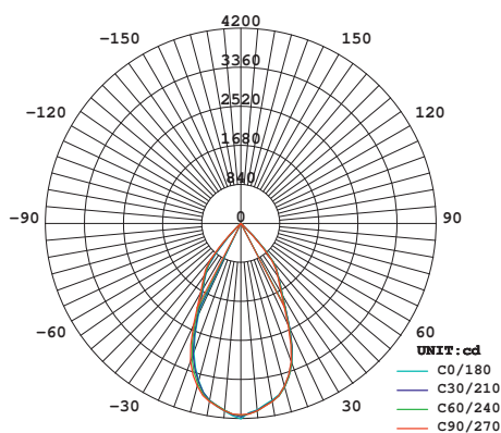
Lichtstärkeverteilung FraR
