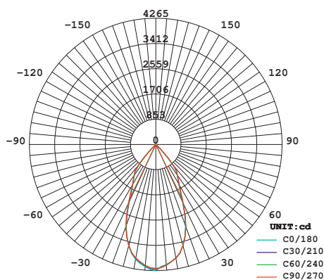
Lichtstärkeverteilung FraS
