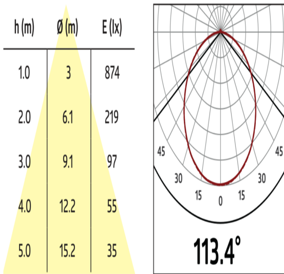
Lichtverteilungskurve
