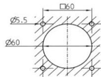
Montageausschnitt
