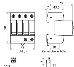
Maßbild DG M TT ACI 385 FM
