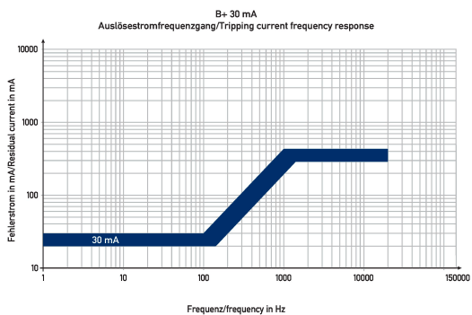
Diagramme FI-/LS-Kombinationen DRCBO 4 C25/0,03/1N-B+
