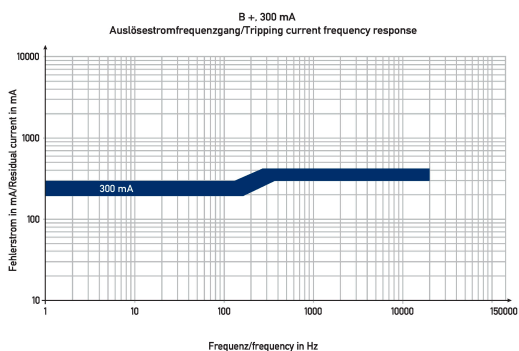
Diagramme FI-/LS-Kombinationen DRCBO 4 C13/0,30/1N-B+
