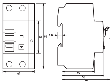
Maßzeichnung FI-/LS-Kombinationen DRCBO 4 C13/0,10/1N-B SK
