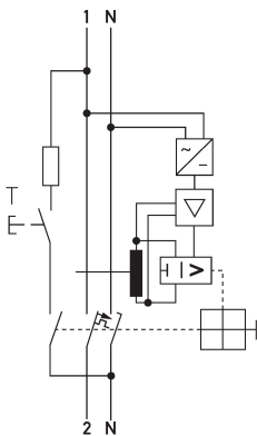
Schaltungsbeispiel FI-/LS-Kombinationen DRCBO 4 B25/0,30/1N-B+
