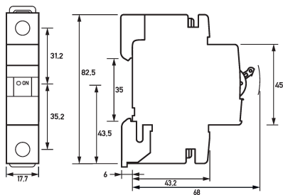
Maßzeichnung Leitungsschutzschalter DLS 6i K3-1
