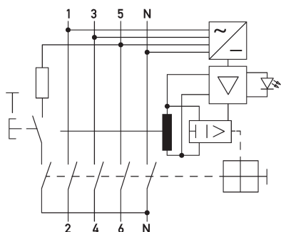
Schaltungsbeispiel Fehlerstromschutzschalter DFS 4 063-4/0,03-B SK R ISO HD
