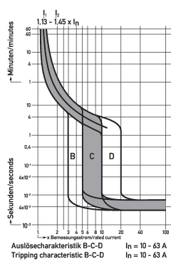
Diagramme Leitungsschutzschalter DLS 6hsl C16-3
