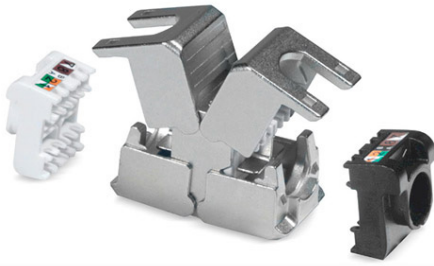
Kabelverbinder Klasse EA, IP20
