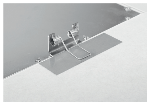
GK-Montage mit SNAP-IN Federeinbausatz für Frame-In-One
