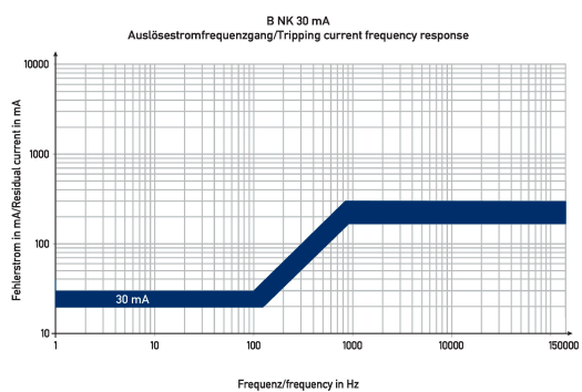
Diagramme FI-/LS-Kombinationen DRCBO 4 Co6/0,03/1N-B NK
